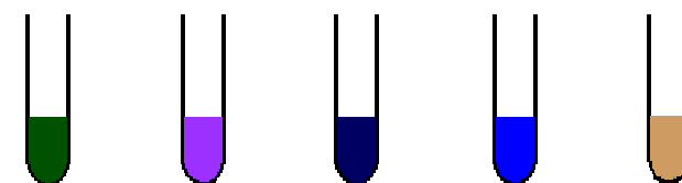
[Cr(OH) 6 ] 3- [Cr(NH 3 ) 6 ] 3+ [Cu(NH 3 ) 4 (H 2 O) 2 ] 2+ [CoCl 4 ] 2- [Co(NH 3 ) 6 ] 2+
