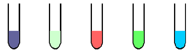
[Cr(H 2 O) 6 ] 3+ [Fe(H 2 O) 6 ] 2+ [Co(H 2 O) 6 ] 2+ [Ni(H 2 O) 6 ] 2+ [Cu(H 2 O) 6 ] 2+
